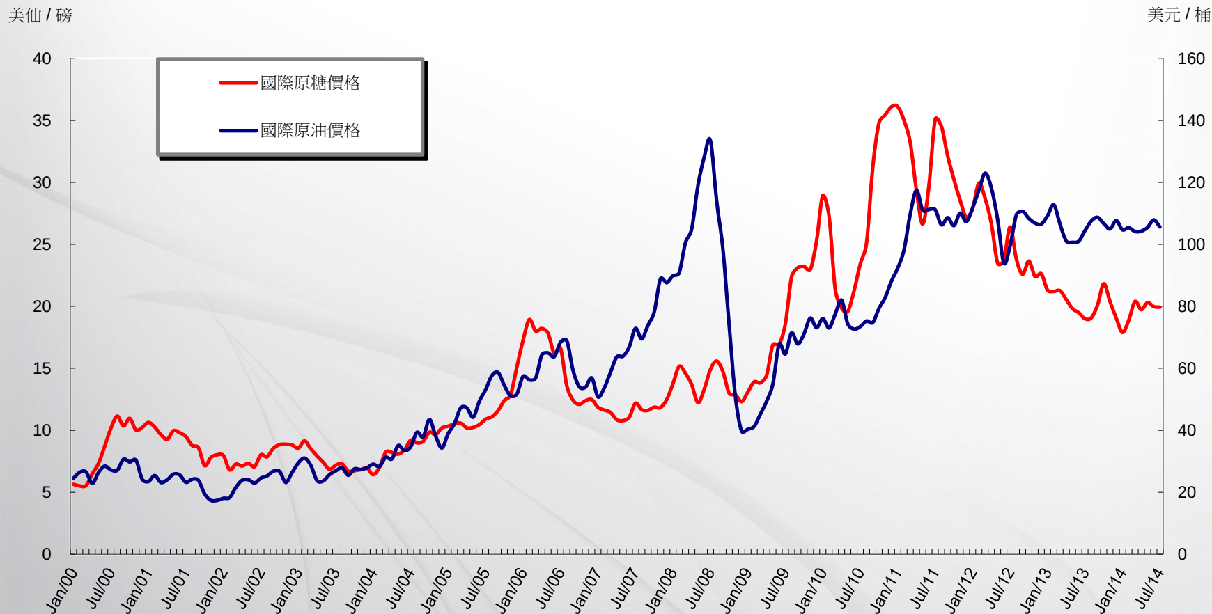
原油價格及糖價關係走勢圖 (2000年1月至2014年 7月)
